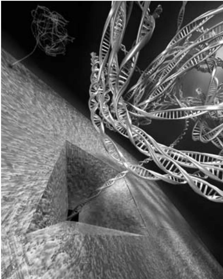
Wetenschappelijke weergave van DNA dat zich verplaatst door een minuscule opening (nanopore) in vaste toestand.
